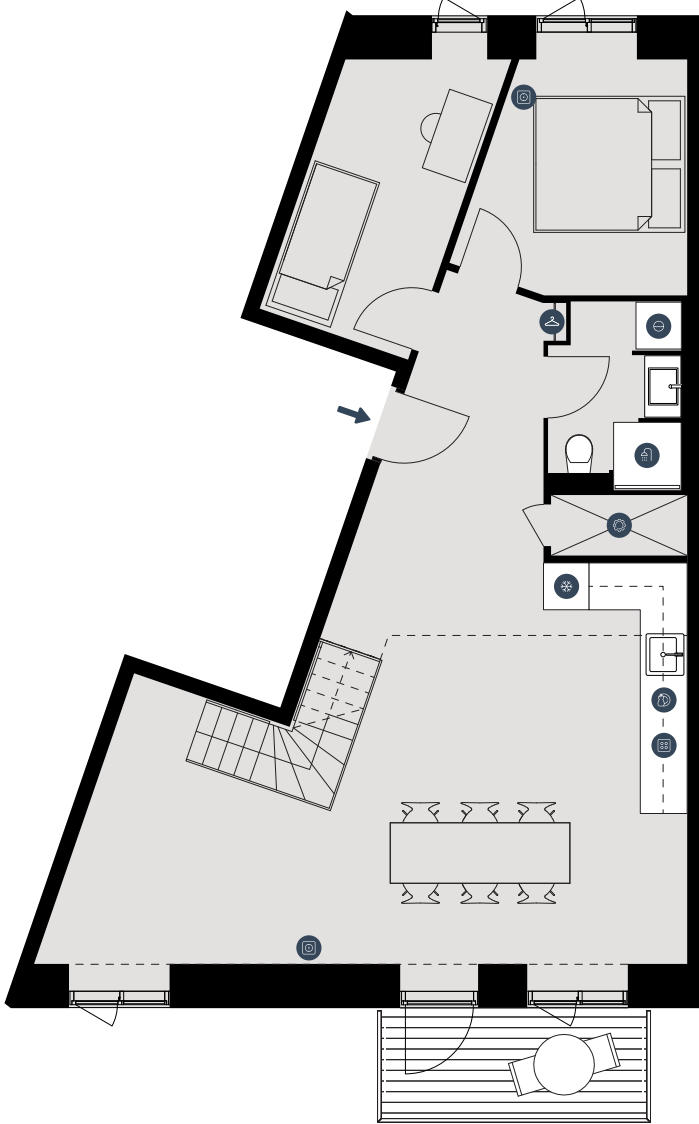
STUEPLAN
