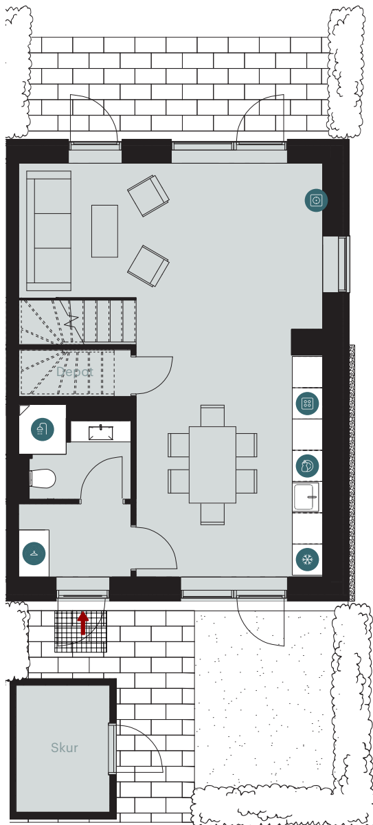
Stueplan
