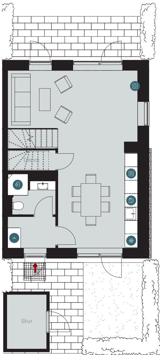
Stueplan
